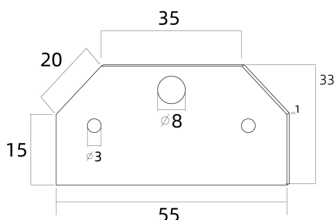
2203-ZP-001 (mm)
