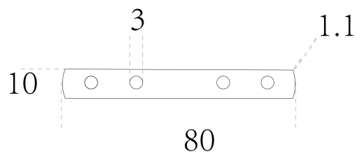
2203-CP-001 (mm)
