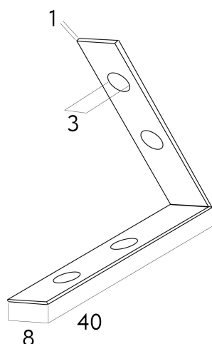
2203-CL-002 (mm)
