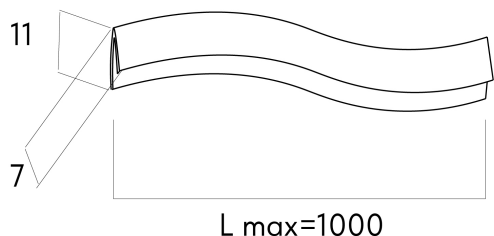
2203-НН-001 (mm)
